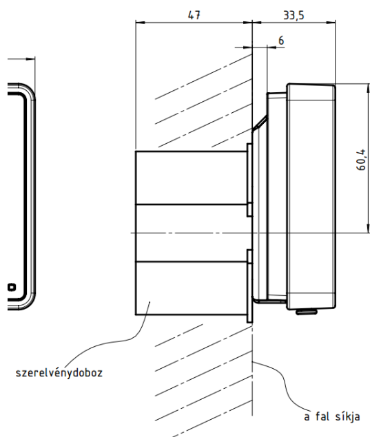
„C” kivitel: szerelvénydobozba illeszkedő, beltéri – spec. kivitel
