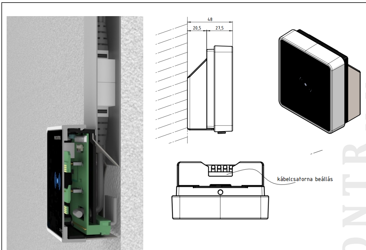
„D” kivitel: kívülről szerelhető, kábelcsatornához javasolt beltéri – spec. kivitel
